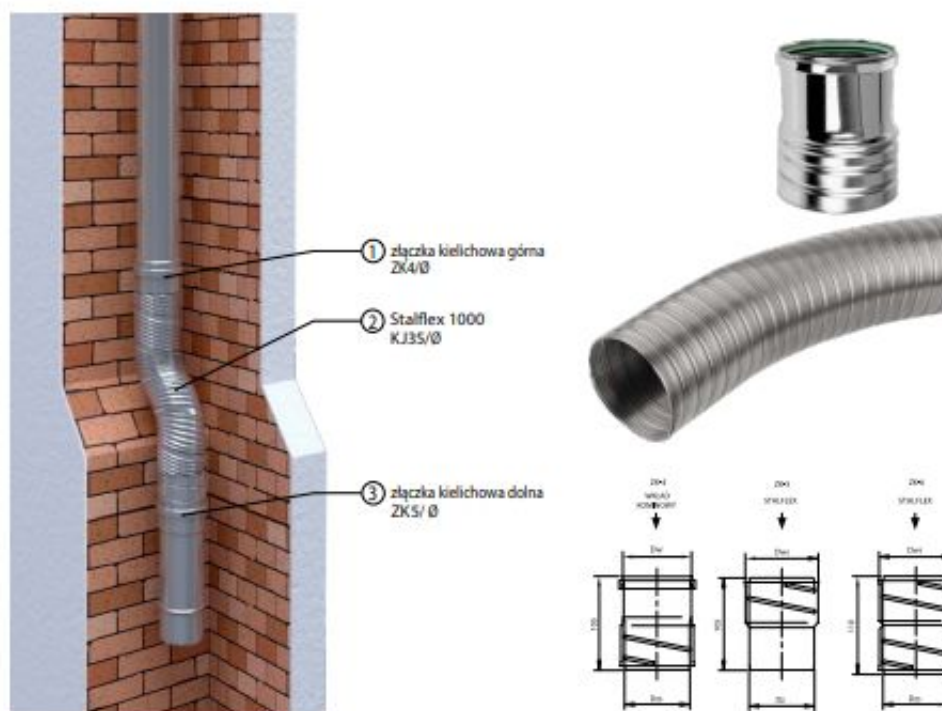
Złączka do połączenia wkładu kominowego z elastycznym przewodem typu stalflex.
