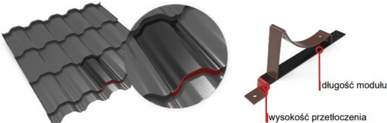
Powyższy schemat obrazuje sposób interpretacji długości modułu oraz wysokości przetłoczenia.
