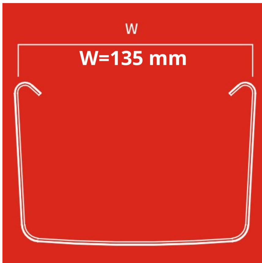
Elementy kwadratowego systemu rynnowego Krop
