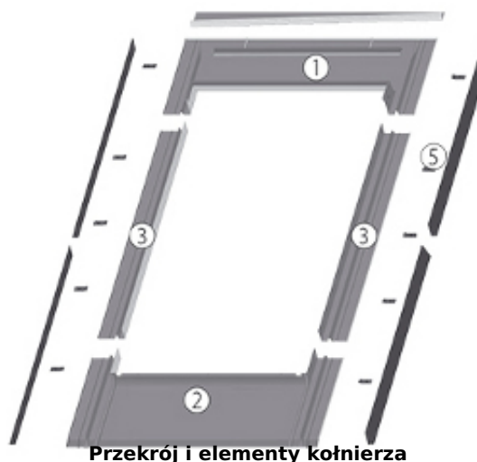
Przekrój i elementy kołnierza
